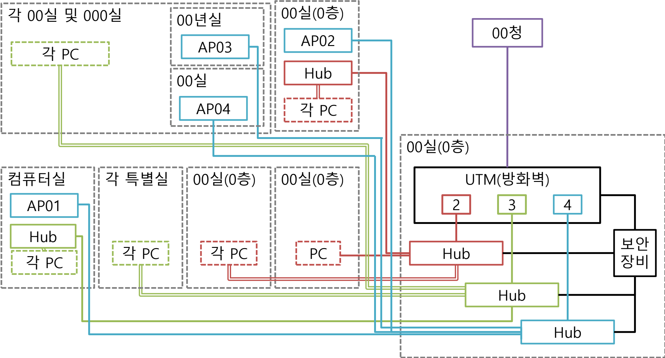
OOOO학교 네트워크 구성도(예시)
