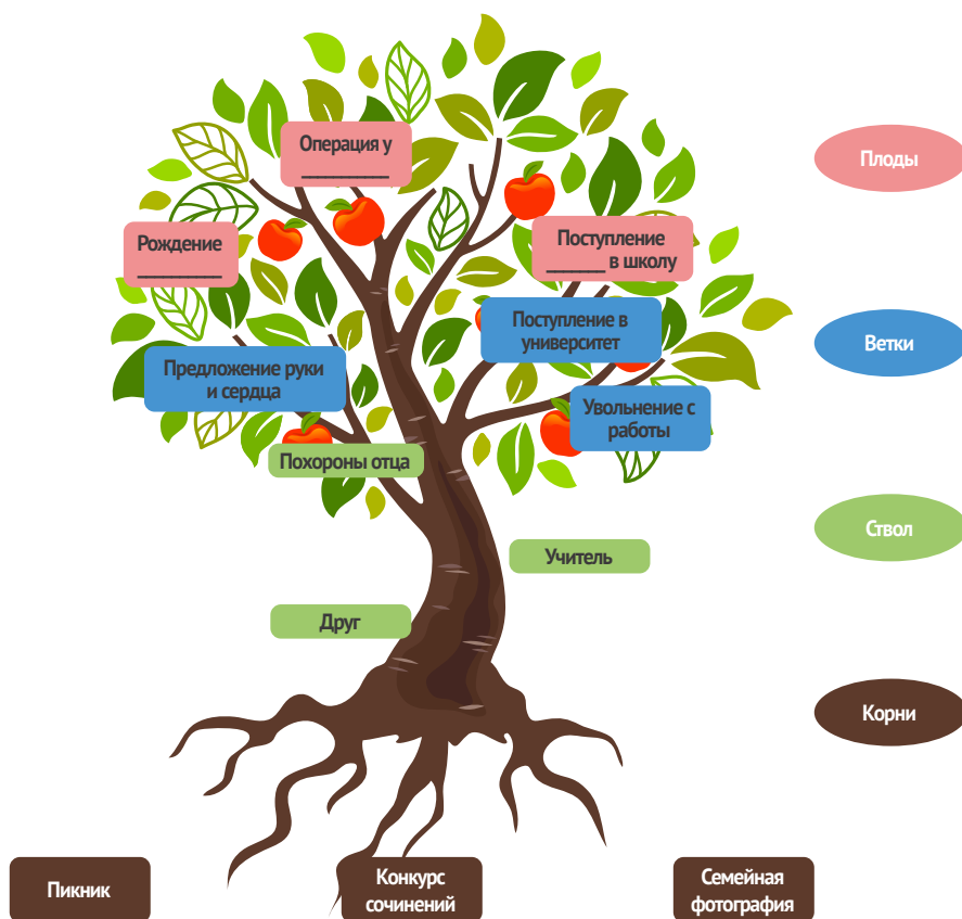
Пример дерева роста
