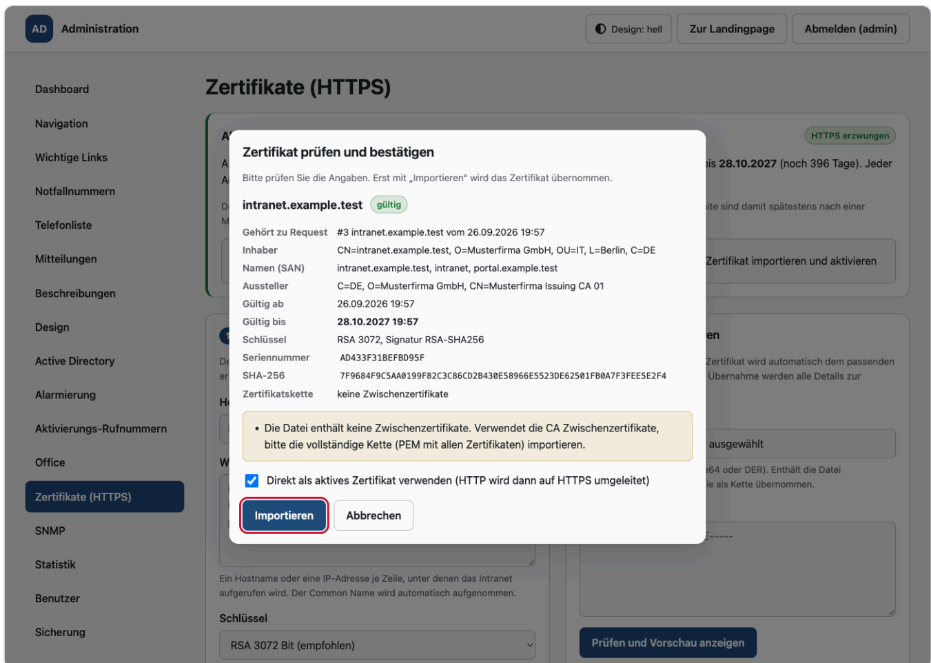
Abb. 17 Vorschau des Zertifikats vor der Übernahme.
