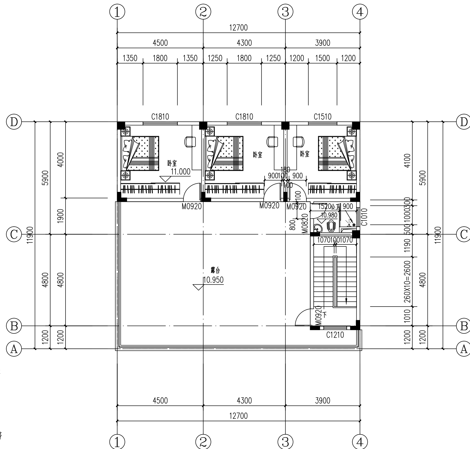
四层平面图 1:100
