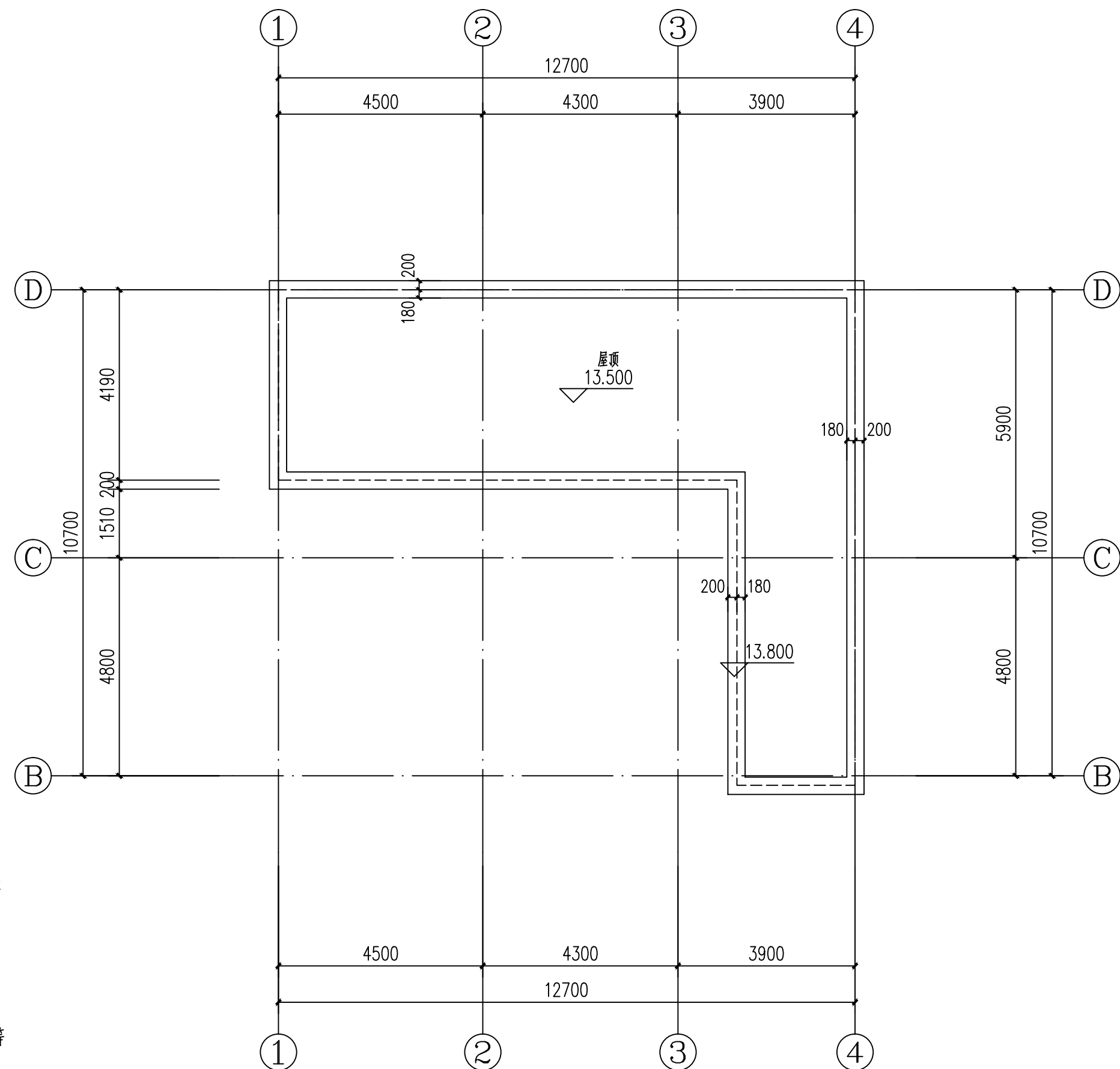
屋顶平面图 1:100
