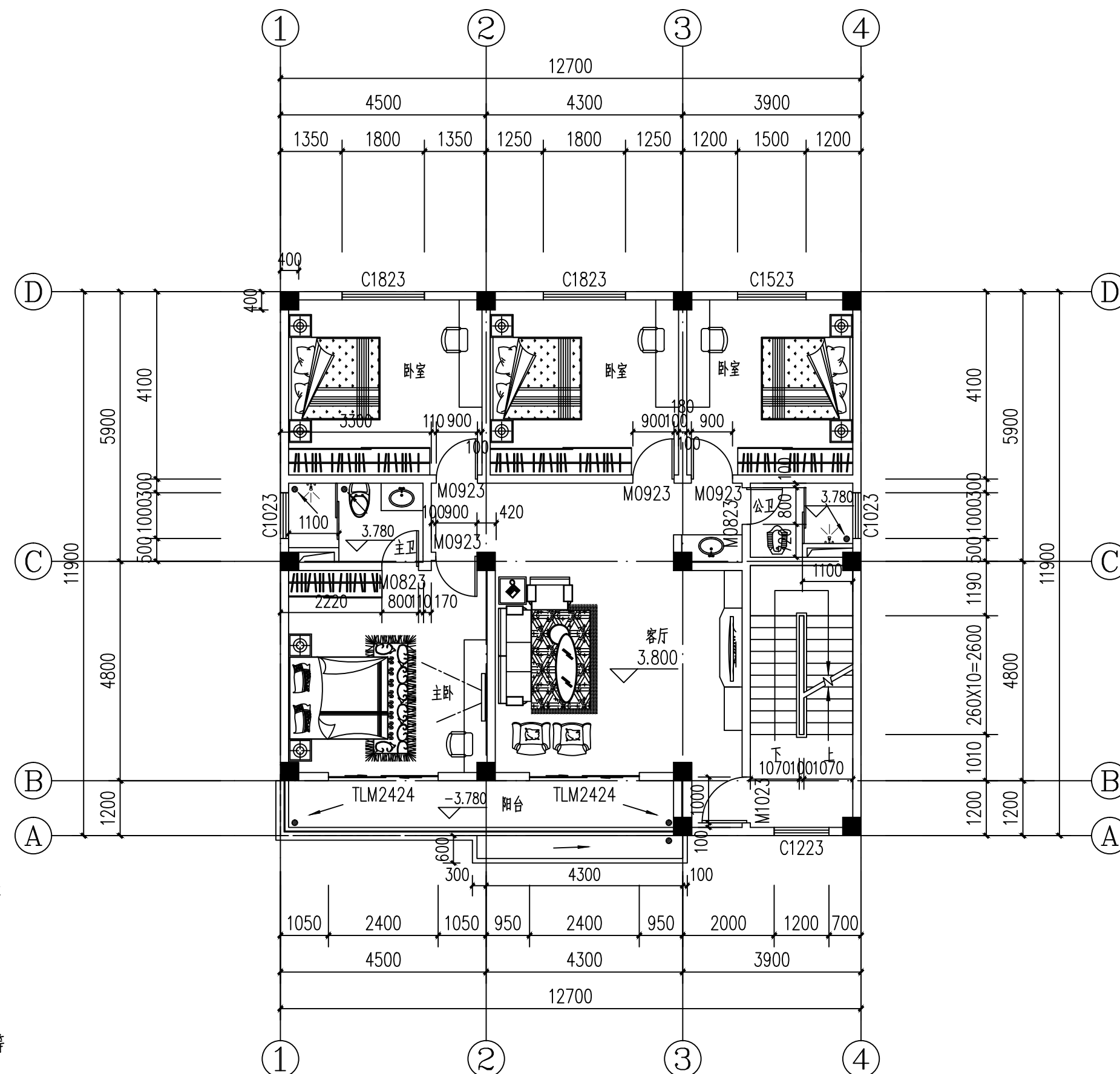
二层平面图 1:100
