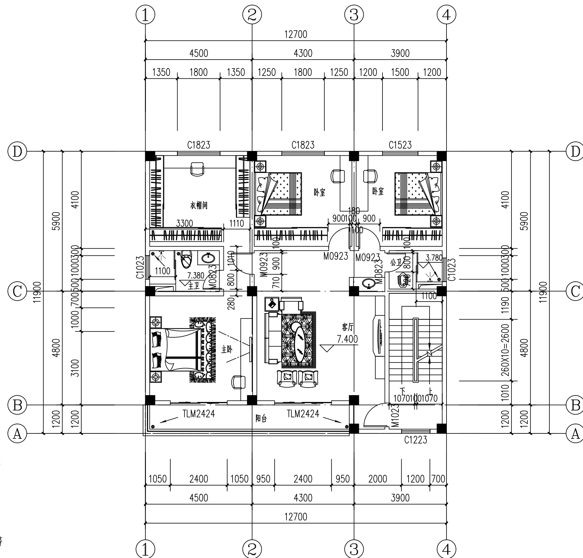
三层平面图 1:100
