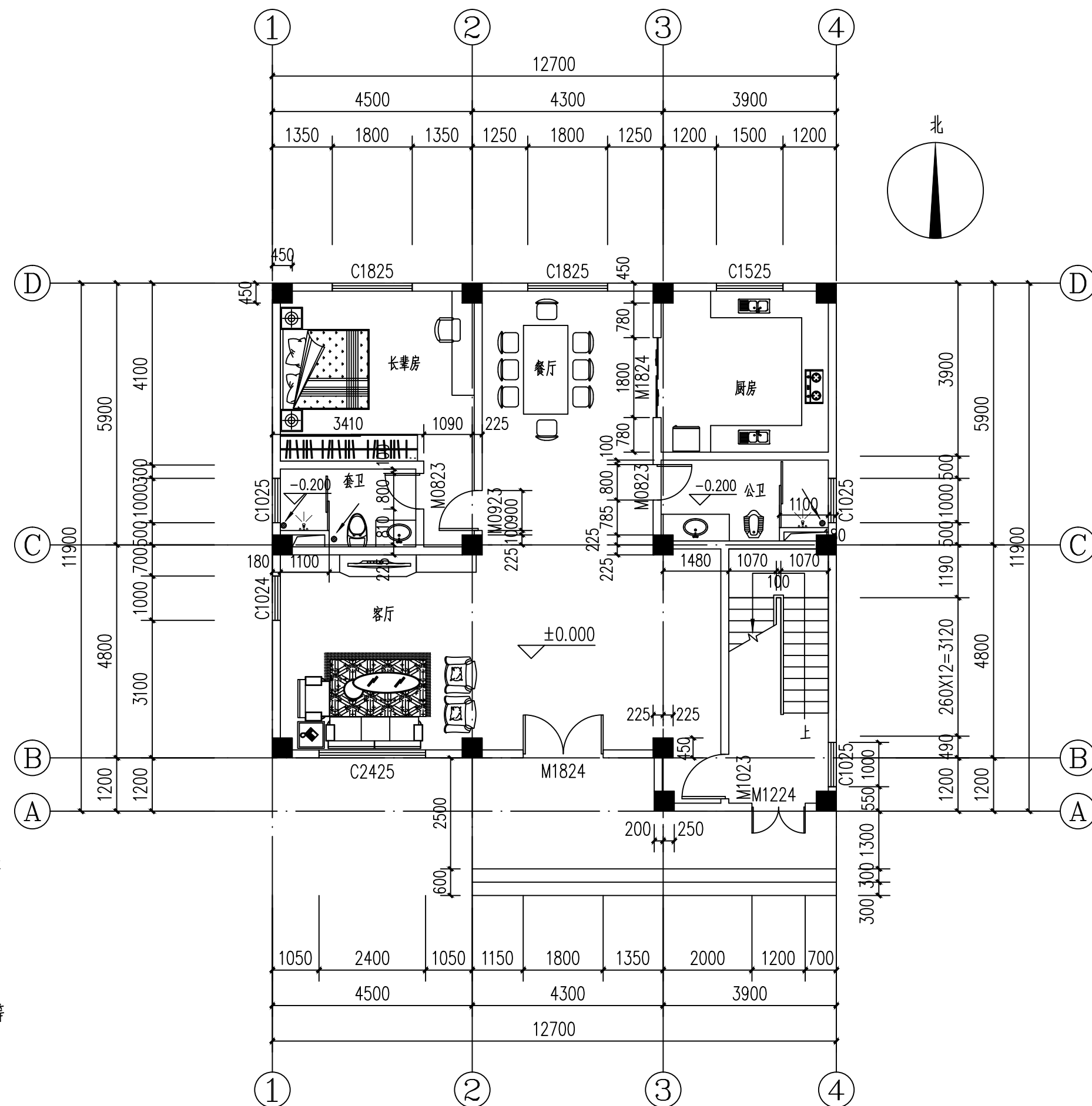
一层平面图 1:100
