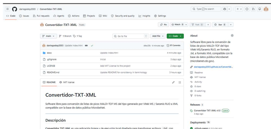
Figura 3. Repositorio Github.
