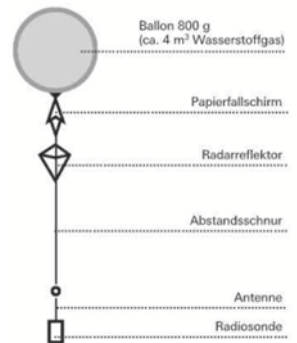
Aufstiegsgerüst für Radiosonden- und Radarwindaufstieg
