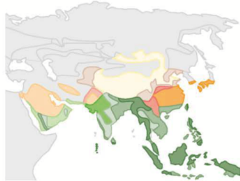
Troll / Paffen
