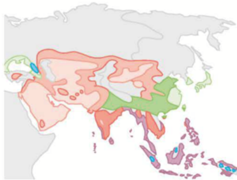
Köppen
