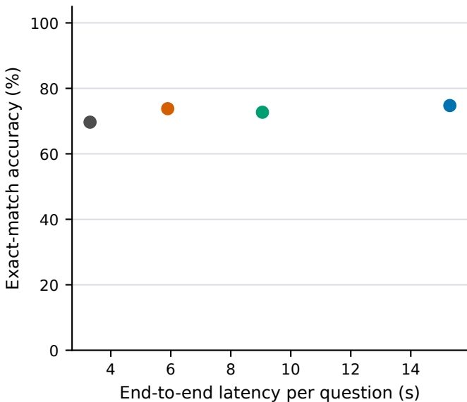
GSM8K
