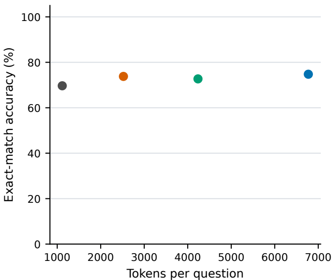
GSM8K
