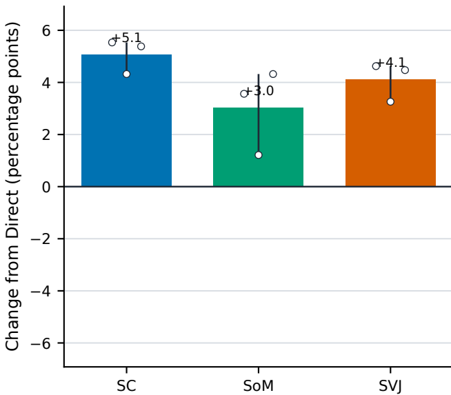
GSM8K
