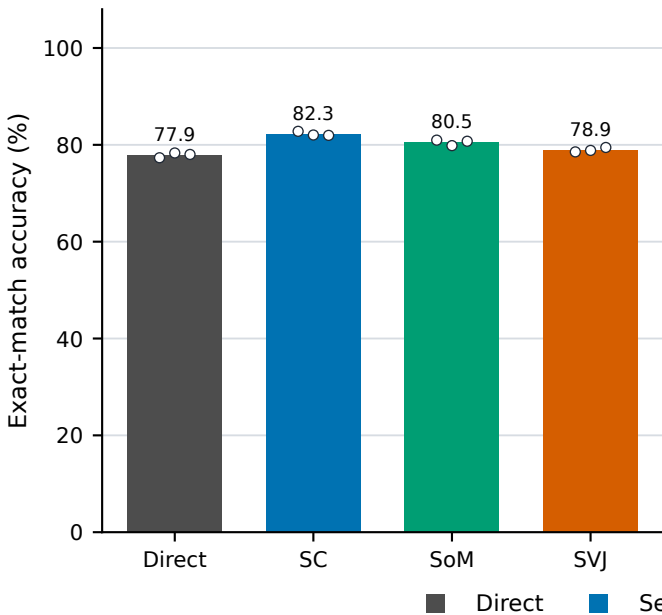
GSM8K
