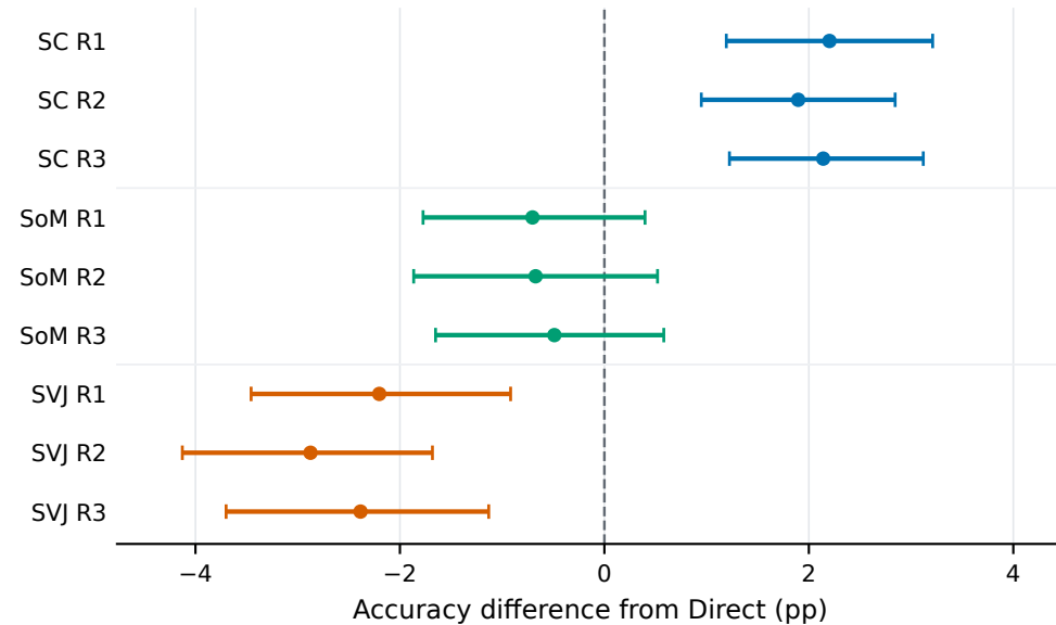
Llama 3.2 3B - BoolQ
