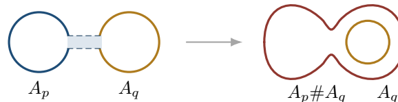
Rysunek 18.4: Schemat przesunięcia w przypadku, gdy sfery przyczepienia są okręgami. Po lewej wybieramy wstęgę między A_p i A_q ; po prawej nowa sfera przyczepienia pierwszego uchwytu przebiega raz także wzdłuż drugiego. Dokładne osadzenie i obramowanie w wyższym wymiarze nie są tu pokazane.
