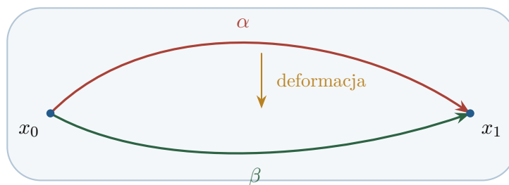
Rysunek 6.1: Homotopia dróg przesuwa ich wnętrza, ale zachowuje oba punkty końcowe.
