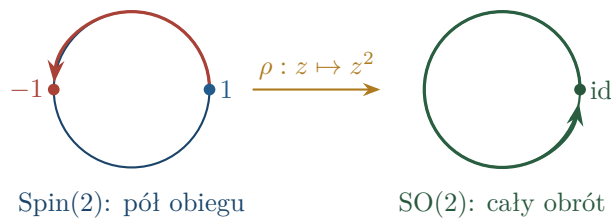
Rysunek 4.4: Droga od 1 do -1 w \text{Spin}(2) rzutuje się na pełen obrót w \text{SO}(2) . Końce drogi są różne w grupie \text{Spin} , choć odpowiadają temu samemu obrotowi.
