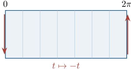
(a) Prostokąt przed sklejeniem
