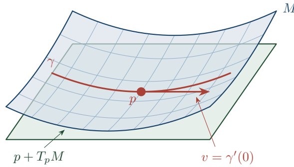
Rysunek 1.10: Przestrzeń styczna: zielony równoległobok przedstawia afiniczną płaszczyznę p + T_p M przy osadzonej powierzchni M . Czerwona krzywa \gamma leży na M , a wektor v = \gamma'(0) leży w płaszczyźnie stycznej. Siatka powierzchni odchyła się od tej płaszczyzny poza punktem p .
