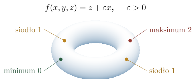
Rysunek 22.3: Torus o przekroju kołowym oglądany ukośnie z góry ( R = 2 , r = 0,69 , \varepsilon = 0,16 ). Znaczniki pokazują rzuty wszystkich czterech punktów krytycznych, także gdy powierzchnia torusa je przesłania. Punkty te mają indeksy 0, 1, 1, 2; składnik \varepsilon x rozdziela ich wartości. Podpoziomice są kolejno dyskiem, pierścieniem, torusem bez dysku i całym torusem.
