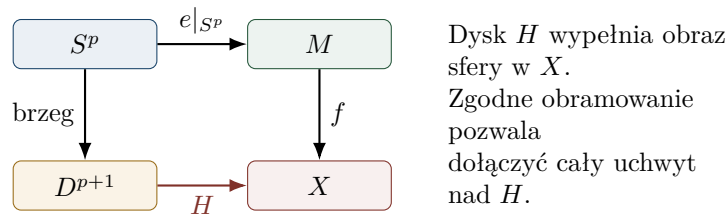
Rysunek 26.4: Warunek na odwzorowanie w kroku chirurgii. Komutatywność diagramu oznacza H|_{S^p} = f \circ e|_{S^p \times \{0\}} . Dodatkowe dane normalne kontrolują obramowanie.
