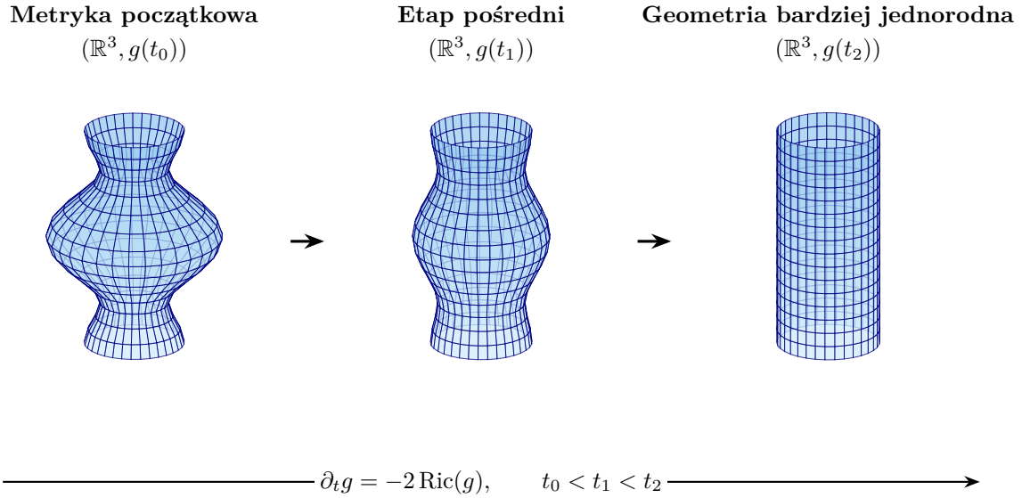
Rysunek 31.1: Schemat ideowy zmiany geometrii na \mathbb{R}^3 w potoku Ricciego \partial_t g = -2 \operatorname{Ric}(g) . Niebieskie powierzchnie siatkowe symbolizują zmniejszanie się wybranej lokalnej deformacji; nie są reprezentacją całej trójwymiarowej metryki. Rysunek nie zakłada, że dowolny potok Ricciego zbiega do metryki euklidesowej.
