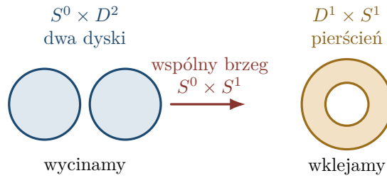
Rysunek 26.1: Lokalny model dla p = 0 , n = 2 . Dwa dyski i pierścień mają ten sam brzeg: dwa okręgi. Ostateczną rozmaitość otrzymujemy, przyklejając pierścień do części starej powierzchni pozostałej po wycięciu dysków. Globalny przykład S^2 \rightarrow T^2 widzieliśmy na Rysunku 23.2.
