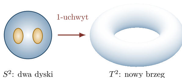
Rysunek 23.2: Dołączenie 1-uchwytu zgodnie z orientacją zmienia brzeg wyjściowy trójwymiarowego kobordyzmu z S^2 na T^2 . Zaznaczone na sferze złote dyski stanowią S^0 \times D^2 ; po wycięciu ich wewnątrz doklejamy pierścień D^1 \times S^1 .
