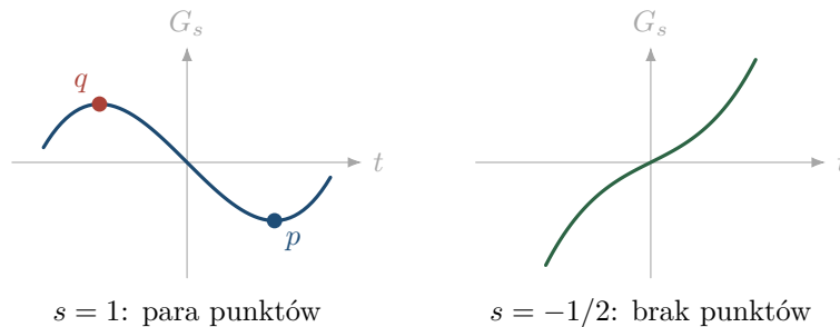
Rysunek 23.5: Przekrój modelu (23.5) przez oś x = y = 0 . Dla s > 0 są dwa punkty krytyczne o kolejnych indeksach i jedna trajektoria od q do p . Po przejściu przez s = 0 oba znikają. Pozostałe kierunki x, y ustalają indeksy.
