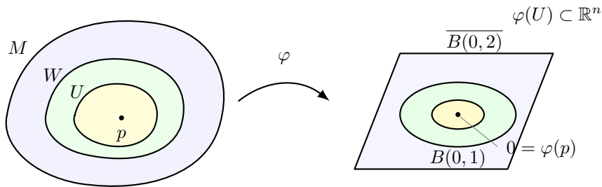
Rysunek 1.8: Wybór mapy (U, \varphi) wokół punktu p : U \subseteq W , \varphi(p) = 0 oraz \overline{B(0, 2)} \subseteq \varphi(U) .
