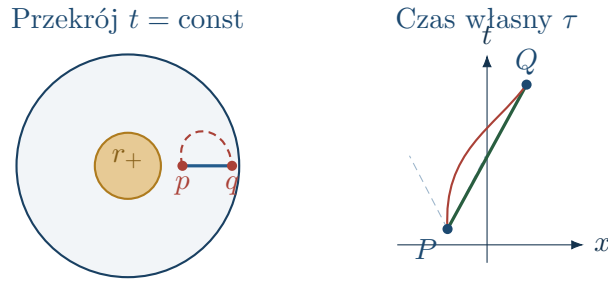
Rysunek 12.9: Po lewej odcinek radialny minimalizuje długość w riemannowskim przekroju przestrzennym. Po prawej prosta czasopodobna maksymalizuje czas własny między ustalonymi zdarzeniami w płaskiej czasoprzestrzeni. Schemat nie przedstawia osadzenia metryki Kerra.
