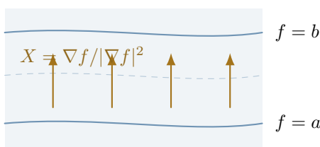
Rysunek 15.4: Przepływ pola X przenosi punkt poziomicy f = a na poziomice f = a + t . Gdy w zwartym pasie nie ma punktów krytycznych, wszystkie poziomice składają się w produkt.
