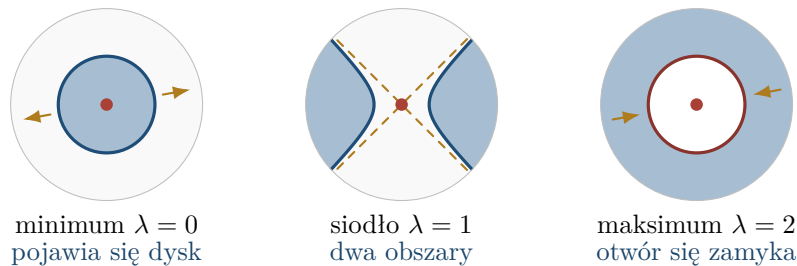
Rysunek 22.1: Lokalne podpoziomice trzech postaci z lematu Morse'a w wymiarze dwa. Kolor niebieski oznacza f \leq a : przy minimum pokazujemy a > f(p) , a przy siodle i maksimum a < f(p) . Żółte strzałki wskazują wzrost f : od minimum na zewnątrz, do maksimum ku środkowi. Przerywane proste przy siodle to poziom krytyczny.
