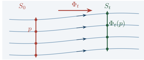
Rysunek 2.2: Przepływ przesuwają punkty wzdłuż krzywych całkowych. Czerwony przekrój poprzeczny S_0 przechodzi w zielony S_t ; oba przekroje mają dokładnie te same wartości stałej y - A \sin(\kappa x) , gdzie A = 0.17 i \kappa = 38\pi/180 . Są to trajektorie pola X = (1, A\kappa \cos(\kappa x)) . Jego przepływ to \Phi_s(x, y) = (x+s, y+A[\sin(\kappa(x+s))-\sin(\kappa x)]) ; na rysunku t = 1.68 - (-1.88) = 3.56 .
