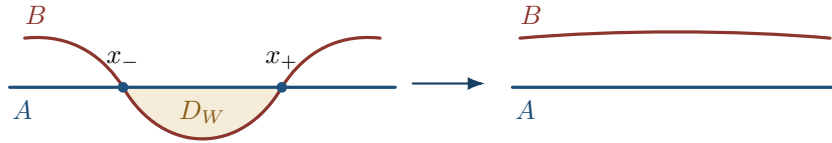
Rysunek 26.5: Przekrój schematyczny ruchu Whitneya. Po lewej łuki na A i B ograniczają jasny dysk, a x_- i x_+ mają przeciwne znaki. Po ruchu przecięć nie ma. Rysunek pokazuje tylko przekrój; w wyższych wymiarach niezbędne jest obramowanie całego dysku.
