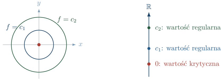
Rysunek 14.1: Dla f(x, y) = x^2 + y^2 punkt krytyczny leży w dziedzinie, a jego wartość krytyczna na osi wyników. Poziomice dodatnie są gładkimi okręgami. Schemat rozróżnia oba pojęcia.
