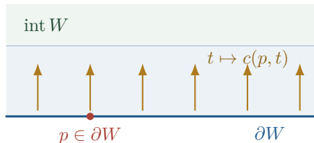
Rysunek 15.3: Kołnierz zamienia całe otoczenie brzegu w produkt \partial W \times [0, 1) . Współrzędna t rośnie do wnętrza rozmaitości.
