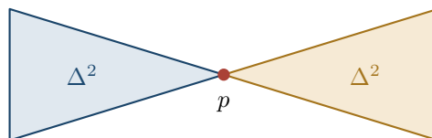
Rysunek 9.5: Dwa trójkąty ze wspólnym wierzchołkiem p . To kompleks symplekjalny, ale w p nie jest powierzchnią gładką, nawet z brzegiem.
