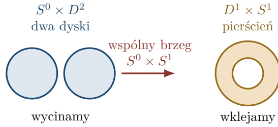
Rysunek 21.1: Lokalny model dla p = 0 , n = 2 . Dwa dyski i pierścień mają ten sam brzeg: dwa okręgi. Ostateczną rozmaitość otrzymujemy, przyklejając pierścień do części starej powierzchni pozostałej po wycięciu dysków. Globalny przykład S^2 \rightarrow T^2 widzieliśmy na Rysunku 18.2.
