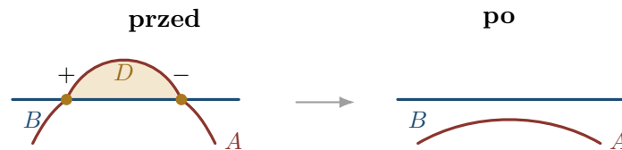
Rysunek 19.3: Dwuwymiarowy przekrój triku Whitneya: punkty o przeciwnych znakach są końcami brzegu złotego dysku D . Przesunięcie czerwonej sfery usuwa oba punkty. Sam dowód działa w poziomicy wymiaru co najmniej 5; rysunek nie przedstawia jej pozostałych wymiarów.
