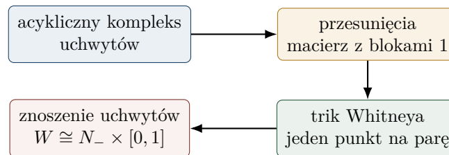
Rysunek 19.1: Cztery etapy dowodu. Acykliczność jest algebraiczna; między nią a zniesieniem uchwytów potrzebne są ruchy geometryczne.
