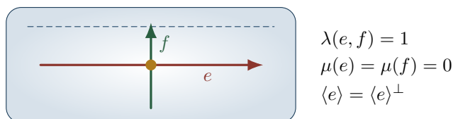
Rysunek 22.1: Lokalny schemat pary hiperbolicznej. Sfery reprezentujące e i f spotykają się poprzecznie w jednym punkcie, a każdą z nich osobno można obramować bez samoprzecięć. Wybór kierunku e wyznacza lagranżjan; prostokąt jest tylko fragmentem otoczenia przecięcia, nie całą rozmaitością.
