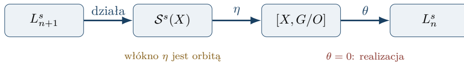
Rysunek 23.1: Środkowa część ciągu chirurgii. Zbiór struktur nie jest zwykle grupą; dokładność opisuje realizowalność normalnych danych oraz orbity działania grupy L_{n+1}^s .
