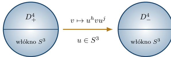
Rysunek 25.1: Schemat sklejania wiązki nad dwiema półsferami S^4 . Kolorowe okręgi oznaczają półsfery w umownym przekroju; zmienna u parametryzuje ich wspólny równik. Mapa na strzałce skręca włókno i określa gładką wiązkę.
