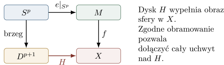
Rysunek 21.3: Warunek na odwzorowanie w kroku chirurgii. Komutatywność diagramu oznacza H|_{S^p} = f \circ e|_{S^p \times \{0\}} . Dodatkowe dane normalne kontrolują obramowanie.
