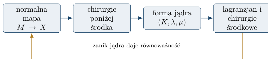
Rysunek 22.2: Kolejne etapy twierdzenia Walla w parzystym wymiarze. Przejście od algebraicznego lagranżjanu do osadzonych sfer wymaga lematów geometrycznych Walla.
