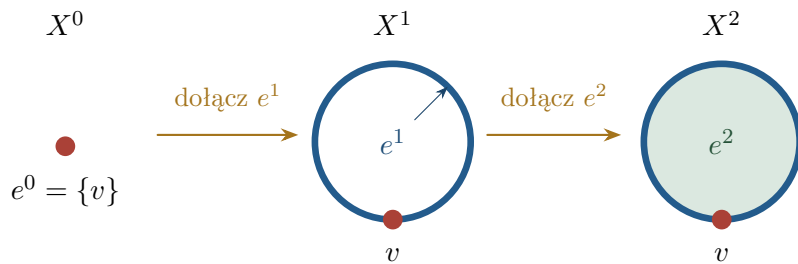
Rysunek 6.5: Przykłady kolejnych wymiarów CW: punkt X^0 = \{v\} , okrąg X^1 \cong S^1 otrzymany przez sklejanie obu końców 1-komórki z v , oraz dysk X^2 \cong D^2 po dołączeniu 2-komórki wzdłuż całego okręgu. Czerwony punkt, niebieski łuk i zielone wnętrze oznaczają odpowiednio otwarte komórki wymiarów 0, 1, 2.
