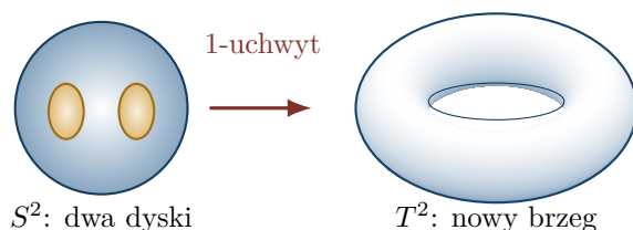
Rysunek 18.2: Dołączenie 1-uchwytu do trójwymiarowego kobordyzmu zmienia jego brzeg z S^2 na T^2 . Zaznaczone na sferze złote dyski stanowią S^0 \times D^2 ; po wycięciu ich wewnątrz doklejamy pierścień D^1 \times S^1 .
