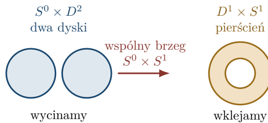
Rysunek 22.1: Lokalny model dla p = 0 , n = 2 . Dwa dyski i pierścień mają ten sam brzeg: dwa okręgi. Ostateczną rozmaitość otrzymujemy, przyklejając pierścień do części starej powierzchni pozostającej po wycięciu dysków. Globalny przykład S^2 \rightarrow T^2 widzieliśmy na Rysunku 19.2.
