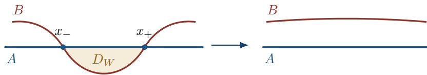
Rysunek 22.4: Przekrój schematyczny ruchu Whitneya. Po lewej łuki na A i B ograniczają jasny dysk, a x_- i x_+ mają przeciwne znaki. Po ruchu przecięć nie ma. Rysunek pokazuje tylko przekrój; w wyższych wymiarach niezbędne jest obramowanie całego dysku.
