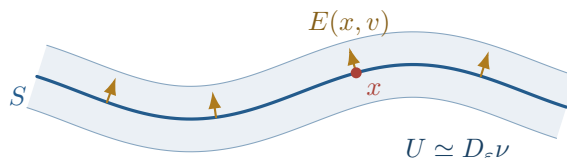
Rysunek 16.2: Otoczenie tubularne krzywej S (ciemnoniebieska). W metryce euklidesowej złote odcinki są prostopadłe do stycznych krzywej, a E(x, v) = x + v umieszcza ich końce w jasnym pasie U . Brzegi pasa są odsunięte wzdłuż normalnych.
