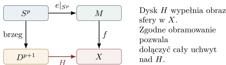
Rysunek 22.3: Warunek na odwzorowanie w kroku chirurgii. Komutatywność diagramu oznacza H|_{S^p} = f \circ e|_{S^p \times \{0\}} . Dodatkowe dane normalne kontrolują obramowanie.
