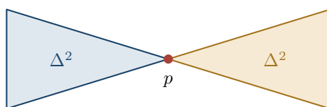
Rysunek 10.5: Dwa trójkąty ze wspólnym wierzchołkiem p . To kompleks symplecjialny, ale w p nie jest powierzchnią gładką, nawet z brzegiem.
