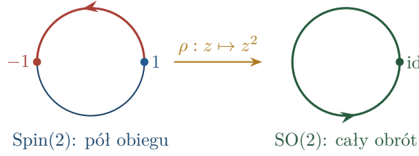
Rysunek 4.4: Droga od 1 do -1 w \text{Spin}(2) rzutuje się na pełen obrót w \text{SO}(2) . Końce drogi są różne w grupie Spin, choć odpowiadają temu samemu obrotowi.
