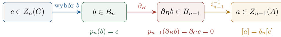
Rysunek 5.1: Odwzorowanie łączące: podnosimy cykl c , bierzemy brzeg podniesienia b , po czym odczytujemy go w A_{n-1} . Odwroćcie i_{n-1} dotyczy tylko jego obrazu \ker p_{n-1} ; całego odwzorowania i_{n-1} nie odwracamy.
