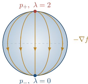
Rysunek 17.4: Spadek funkcji wysokości na sferze. Dla metryki indukowanej trajektorie są południkami i biegną od maksimum do minimum; rysunek pokazuje ich rzuty. Południowy punkt jest stabilny w dwóch wymiarach, a północny niestabilny w dwóch wymiarach; pozostałe zbiory stabilne lub niestabilne tych punktów to same punkty.
