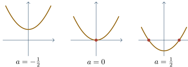
Rysunek 14.3: Poziom zero rodziny F_a(t) = t^2 - a . Zmiana parametru rozбивa styczność w dwa przecięcia transwersalne albo usuwa przecięcie; sam parametr a = 0 jest wyjątkowy.
