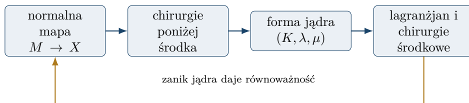
Rysunek 23.2: Kolejne etapy twierdzenia Walla w parzystym wymiarze. Przejście od algebraicznego lagranżjanu do osadzonych sfer wymaga lematów geometrycznych Walla.
