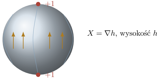
Rysunek 16.4: Gradient wysokości na S^2 ma dwa zera: na biegunie dolnym i górnym. Oba mają indeks +1 , więc suma indeksów i \chi(S^2) są równe 2.
