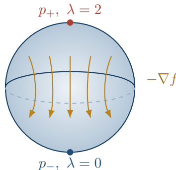
Rysunek 17.4: Spadek funkcji wysokości na sferze. Trajektorie biegną od maksimum do minimum. Południowy punkt jest stabilny w dwóch wymiarach, a północny niestabilny w dwóch wymiarach; pozostałe zbiory stabilne lub niestabilne tych punktów to same punkty.
