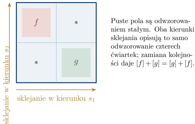
Rysunek 8.1: Dwa niezależne kierunki sklejania w \pi_2 . W \pi_n dla n \geq 2 pozostałe współrzędne traktujemy jako parametry.
