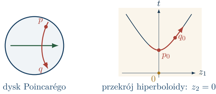
Rysunek 13.5: Po lewej geodezyjne dysku: średnica i łuk okręgu prostopadłego do brzegu (końce na brzegu nie należą do geodezyjnej). Po prawej dokładny przekrój hiperboloidy t^2 - z_1^2 - z_2^2 = 1 , t > 0 , płaszczyzną liniową z_2 = 0 . Czerwona geodezyjna ma postać (\cosh u, \sinh u, 0) ; zaznaczono p_0 dla u = 0 i q_0 dla u = 1 . Płaszczyzna przekroju zawiera początek 0.
