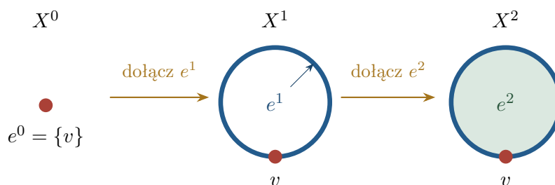
Rysunek 7.5: Przykłady kolejnych wymiarów CW: punkt X^0 = \{v\} , okrąg X^1 \cong S^1 otrzymany przez sklejanie obu końców 1-komórki z v , oraz dysk X^2 \cong D^2 po dołączeniu 2-komórki wzdłuż całego okręgu. Czerwony punkt, niebieski łuk i zielone wnętrze oznaczają odpowiednio otwarte komórki wymiarów 0, 1, 2.
