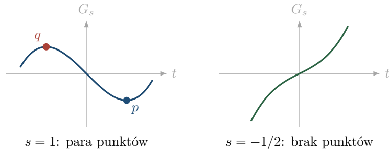
Rysunek 19.5: Przekrój modelu (19.5) przez oś x = y = 0 . Dla s > 0 są dwa punkty krytyczne o kolejnych indeksach i jedna trajektoria od q do p . Po przejściu przez s = 0 oba znikają. Pozostałe kierunki x, y ustalają indeksy.
