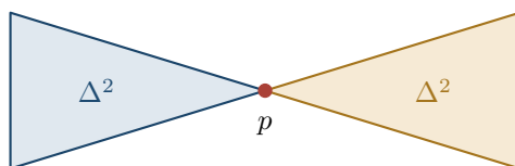
Rysunek 10.5: Dwa trójkąty ze wspólnym wierzchołkiem p . To kompleks symplecjalny, ale w p nie jest powierzchnią gładką, nawet z brzegiem.
