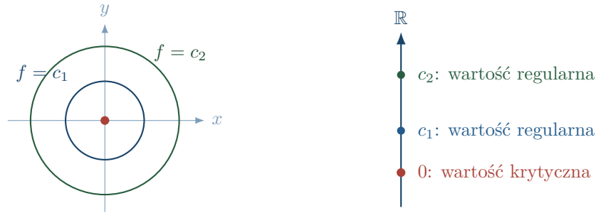
Rysunek 15.1: Dla f(x, y) = x^2 + y^2 punkt krytyczny leży w dziedzinie, a jego wartość krytyczna na osi wyników. Poziomice dodatnie są gładkimi okręgami. Schemat rozróżnia oba pojęcia.
