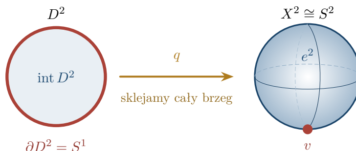
Rysunek 7.6: Struktura CW sfery: D^2 dołączamy do punktu v odwzorowaniem stałym na całym brzegu; q : D^2 \rightarrow D^2 / \partial D^2 jest mapą ilorazową. W powstałej sferze czerwony punkt to jedyne e^0 , a cała pozostała powierzchnia to jedna otwarta komórka e^2 . Nie występują komórki wymiaru 1.
