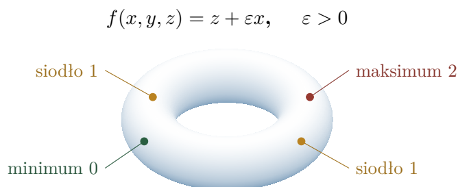
Rysunek 18.3: Torus o przekroju kołowym oglądany ukośnie z góry ( R = 2 , r = 0,69 , \varepsilon = 0,16 ). Znaczniki pokazują rzuty wszystkich czterech punktów krytycznych, także gdy powierzchnia torusa je przesłania. Punkty te mają indeksy 0, 1, 1, 2; składnik \varepsilon x rozdziela ich wartości. Podpoziomice są kolejno dyskiem, pierścieniem, torusem bez dysku i całym torusem.
