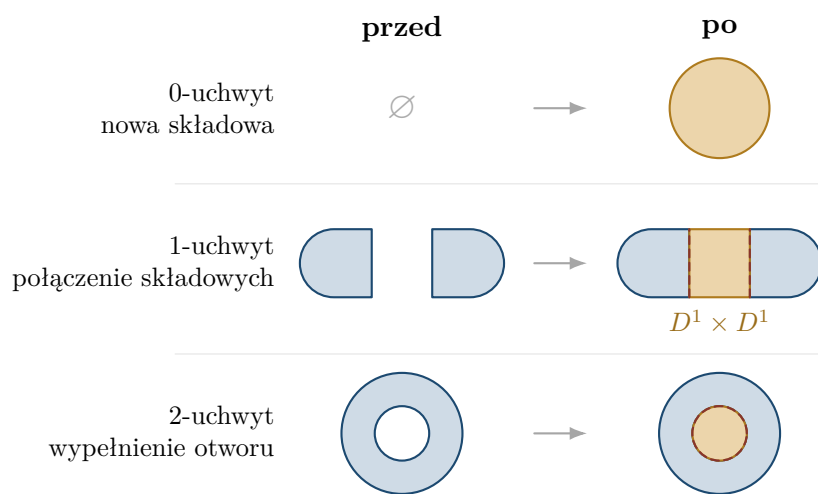
Rysunek 18.2: Trzy niezależne przykłady dla dwuwymiarowej podpoziomicy, pokazane z góry. Niebieski oznacza część istniejącą, złoty nowy uchwyt, a czerwone przerywane odcinki lub okrąg — część przyczepianą. W drugim wierszu prostokąt przykleja się dokładnie do dwóch odcinków brzegu. Inne przyklejenie 1-uchwytu może utworzyć otwór zamiast połączyć składowe.
