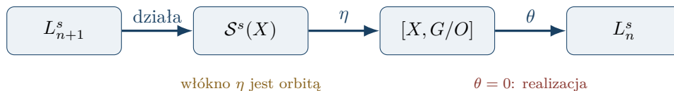
Rysunek 24.1: Środkowa część ciągu chirurgii. Zbiór struktur nie jest zwykłą grupą; dokładność opisuje realizowalność normalnych danych oraz orbity działania grupy L_{n+1}^s .
