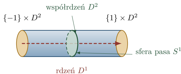
Rysunek 23.1: Uchwyty indeksu 1 w trójwymiarowym kobordyzmie: dwie złote podstawy są przyczepiane do starego brzegu. Czerwona przerywana oś jest rdzeniem; zielony środkowy dysk jest współrdzeniem, a jego okrąg brzegowy to sfera pasa. Rysunek pokazuje sam uchwyt, bez reszty kobordyzmu.
