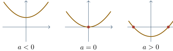
Rysunek 14.3: Poziom zero rodziny F_a(t) = t^2 - a . Zmiana parametru rozbija styczność w dwa przecięcia transversalne albo usuwa przecięcie; sam parametr a = 0 jest wyjątkowy.
