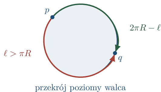
Rysunek 13.5: Ten sam okrąg oglądany jako poziomy przekrój płaskiego walca. Między p i q dłuższy łuk (czerwony) jest geodezyjną bez punktów sprzężonych, lecz krótszy łuk (zielony) wygrywa globalnie.
