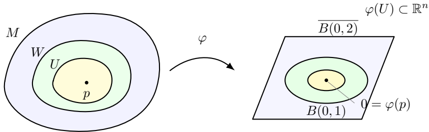
Rysunek 1.8: Wybór mapy (U, \varphi) wokół punktu p : U \subseteq W , \varphi(p) = 0 oraz \overline{B(0, 2)} \subseteq \varphi(U) .
