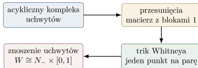
Rysunek 24.1: Cztery etapy dowodu. Acykliczność jest algebraiczna; między nią a zniesieniem uchwytów potrzebne są ruchy geometryczne.
