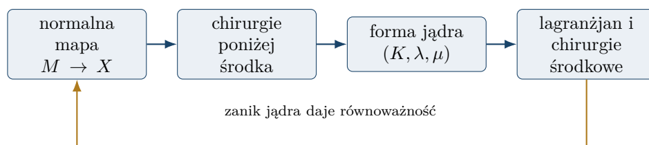
Rysunek 27.3: Kolejne etapy twierdzenia Walla w parzystym wymiarze. Przejście od algebraicznego lagranżjanu do zanurzonych sfer wymaga lematów geometrycznych Walla.
