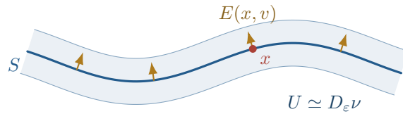
Rysunek 20.2: Otoczenie tubularne krzywej S (ciemnoniebieska). W metryce euklidesowej złote odcinki są prostopadłe do stycznych krzywej, a E(x, v) = x + v umieszcza ich końce w jasnym pasie U . Brzegi pasa są odsunięte wzdłuż normalnych.
