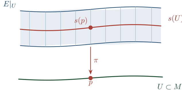
Rysunek 1.13: Sekcja s wybiera dokładnie jeden wektor s(p) w każdym włóknie nad p . Czerwona krzywa przedstawia jej obraz nad pokazanym fragmentem U .
