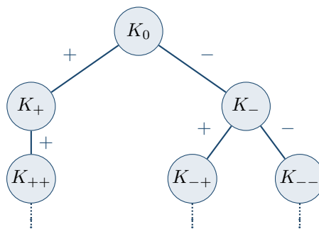
Rysunek 35.1: Pierwsze trzy poziomy drzewa. K_0 ma dwa załamania o znakach + i - ; dlatego w drugim piętrze są dwa uchwyty. Ich załamania wyznaczają trzecie piętro. Kropki oznaczają dalsze poziomy, a nie końcowe wierzchołki.
