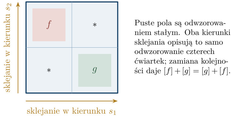
Rysunek 9.1: Dwa niezależne kierunki sklejenia w \pi_2 . W \pi_n dla n \geq 2 pozostałe współrzędne traktujemy jako parametry.
