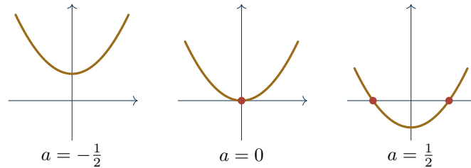
Rysunek 19.3: Poziom zero rodziny F_a(t) = t^2 - a . Zmiana parametru rozбивa styczność w dwa przecięcia transwersalne albo usuwa przecięcie; sam parametr a = 0 jest wyjątkowy.
