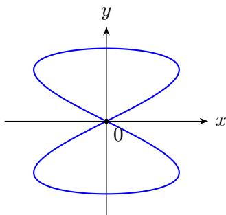
Rysunek 1.16: Krzywa ósemkowa \beta(t) = (\sin 2t, \sin t) : różnowartościowa immersja, która nie jest zanurzeniem — oba końce ( t \rightarrow \pm\pi ) zbiegają do początku układu współrzędnych.
