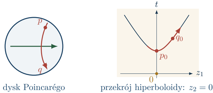
Rysunek 13.5: Po lewej geodezyjne dysku: średnica i łuk okręgu prostopadłego do brzegu (końce na brzegu nie należą do geodezyjnej). Po prawej dokładny przekrój hiperboloidy t^2 - z_1^2 - z_2^2 = 1 , t > 0 , płaszczyzną liniową z_2 = 0 . Czerwona geodezyjna ma postać (\cosh u, \sinh u, 0) ; zaznaczono p_0 dla u = 0 i q_0 dla u = 1 . Płaszczyzna przekroju zawiera początek 0.
