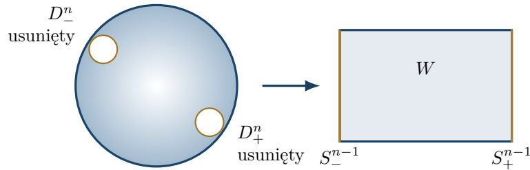
Rysunek 29.1: Schemat wycięcia dwóch dysków z \Sigma^n . Prostokąt przedstawia kobordyzm po zastosowaniu twierdzenia o h -kobordyzmie; dla n \geq 6 jest on gładkim iloczynem. Rysunek jest schematyczny, nie jest zanurzeniem \Sigma^n w płaszczyźnie.
