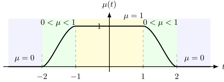
Rysunek 1.9: Jednowymiarowy przekrój funkcji odcinającej \mu . Funkcja jest równa 1 dla |t| \leq 1 , płynnie maleje dla 1 < |t| < 2 i znika dla |t| \geq 2 .
