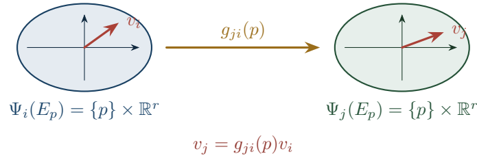
Rysunek 1.15: Dwie trywializacje tego samego włókna E_p . Wektor e ma współrzędne v_i i v_j , związane macierzą przejścia g_{ji}(p) .
