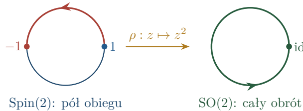
Rysunek 4.4: Droga od 1 do -1 w \mathrm{Spin}(2) rzutuje się na pełen obrót w \mathrm{SO}(2) . Końce drogi są różne w grupie \mathrm{Spin} , choć odpowiadają temu samemu obrotowi.
