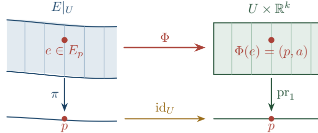
Rysunek 1.12: Trywializacja \Phi: E|_U \rightarrow U \times \mathbb{R}^k jest liniowa na włóknach i zachowuje punkt bazy: \text{pr}_1 \circ \Phi = \pi . Linie przedstawiają włókna schematycznie.
