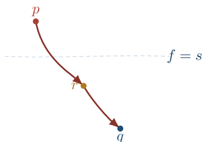
Rysunek 22.5: Schemat trajektorii łamanej p \rightarrow r \rightarrow q . Pojedyncza trajektoria od p do q może się do niej zbliżać, spędzając coraz więcej czasu blisko r . Taka granica jest punktem brzegowym jednowymiarowej przestrzeni trajektorii, gdy różnica indeksów p, q wynosi 2.
