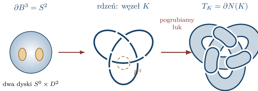
Rysunek 26.2: Przestrzenny przykład operacji z Rysunku 26.1. Najpierw zaznaczamy dwa dyski na sferze. W środku widać rzut węzła trójlistnego; białe przerwy oznaczają przejścia pod spodem, a złoty okrąg małą kulę wokół fragmentu rdzenia. Po prawej pogrubiona pozostała część węzła jest 1-uchwytem przyklejonym do kuli; jej brzeg to zawężony torus.
