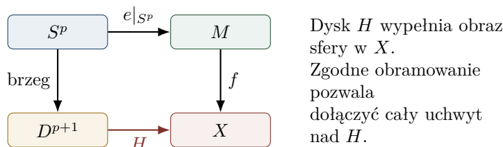
Rysunek 26.4: Warunek na odwzorowanie w kroku chirurgii. Komutatywność diagramu oznacza H|_{S^p} = f \circ e|_{S^p \times \{0\}} . Dodatkowe dane normalne kontrolują obramowanie.
