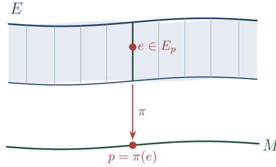
Rysunek 1.11: Lokalny obraz wiązki \pi: E \rightarrow M . Wyróżniono wektor e i jego rzut \pi(e) = p . Włókna narysowano jako fragmenty prostych; ogólnie mają wymiar k .
