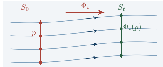
Rysunek 2.2: Przepływ przesuwają punkty wzdłuż krzywych całkowych. Czerwony przekrój poprzeczny S_0 przechodzi w zielony S_t ; oba przekroje mają dokładnie te same wartości stałej y - A \sin(\kappa x) , gdzie A = 0.17 i \kappa = 38\pi/180 . Są to trajektorie pola X = (1, A\kappa \cos(\kappa x)) . Jego przepływ to \Phi_s(x, y) = (x+s, y+A[\sin(\kappa(x+s))-\sin(\kappa x)]) ; na rysunku t = 1.68 - (-1.88) = 3.56 .
