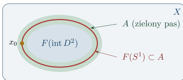
Rysunek 9.2: Przykład odwzorowania względnego (D^2, S^1, *) \rightarrow (X, A, x_0) . Czerwony obraz brzegu leży w zielonym pasie A , podczas gdy obraz wnętrza dysku może wyjść poza A . W ogólnej definicji nie wymaga się różnowartościowości F .
