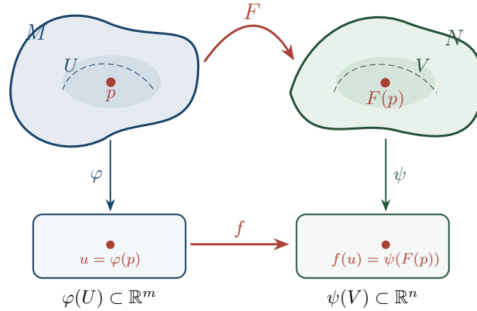
Rysunek 1.4: Odwzorowanie F: M \rightarrow N oraz jego lokalny zapis współrzędnościowy. Po wybraniu map (U, \varphi) i (V, \psi) gładkość F bada się poprzez zwykłe odwzorowanie \psi \circ F \circ \varphi^{-1} między otwartymi podzbiórami przestrzeni euklidesowych.
