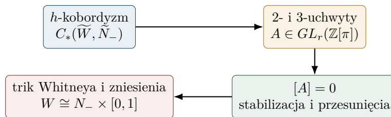
Rysunek 25.2: Logika dowodu twierdzenia o s -kobordyzmie. Acykliczność daje odwracalność A ; znikanie jej klasy w grupie Whiteheada daje dopuszczalną redukcję do I . Na końcu potrzebny jest jeszcze geometryczny trik Whitneya.
