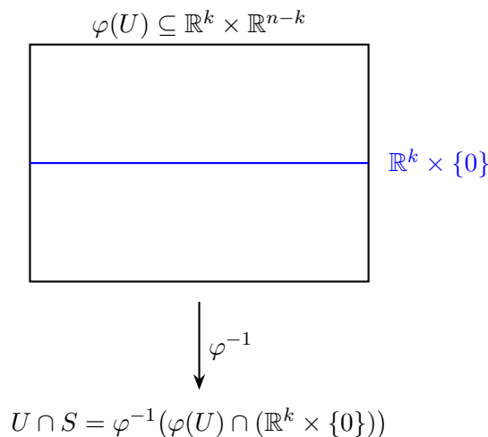
Rysunek 1.17: Mapa plasterkowa: w mapie \varphi , przecięcie U \cap S odpowiada dokładnie przecięciu \varphi(U) z podprzestrzenią \mathbb{R}^k \times \{0\} .
