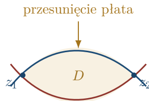
Rysunek 15.1: Schemat dysku Whitneya D : dwa łuki jego brzegu leżą na różnych płatach immersji i łączą dwa punkty podwójne z_1, z_2 . Ruch płata po dysku usuwa oba przecięcia, gdy obramowanie brzegowe da się przedłużyć na D . Rysunek pokazuje tylko dwuwymiarowy przekrój konstrukcji.
