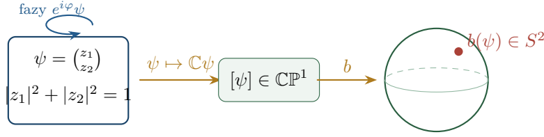
Rysunek 4.5: Spinor jednostkowy \psi \in \mathbb{C}^2 ma fazę, która nie zmienia prostej [\psi] \in \mathbb{CP}^1 . Wzór (4.12) przypisuje tej prostej punkt sfery. To łączy spinory z grassmannianem prostych.
