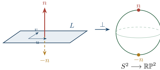
Rysunek 4.2: Orientacja płaszczyzny w \mathbb{R}^3 wybiera jedną z dwóch jednostkowych normalnych. Zapomnienie orientacji utożsamia punkty antypodyczne n i -n na sferze.
