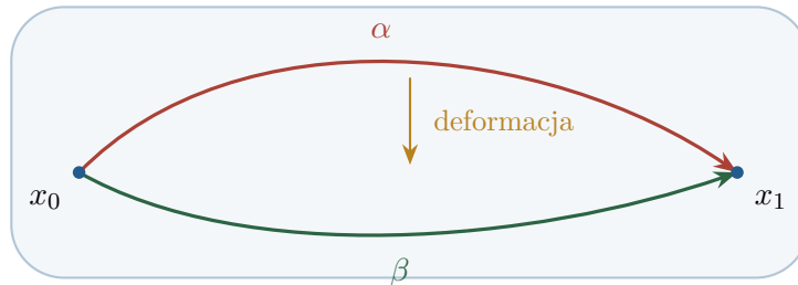
Rysunek 6.1: Homotopia dróg przesuwająca ich wnętrza, ale zachowująca oba punkty końcowe.
