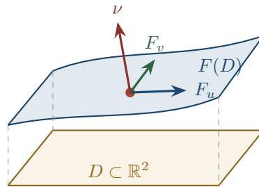
Rysunek 10.2: Parametryzacja unosi obszar parametrów D na powierzchnię. Wektory F_u, F_v wyznaczają element pola \sqrt{\det(g(F_a, F_b))} du dv ; normalna \nu pozwala dodatkowo mierzyć strumień.
