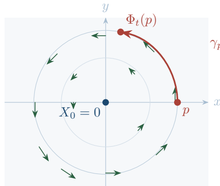
Rysunek 2.2: Pole obrotowe X = (-y, x) : zielone strzałki są wartościami pola, a czerwona krzywa jest jego krzywą całkową. Strzałka pola w każdym punkcie jest styczna do trajektorii.
