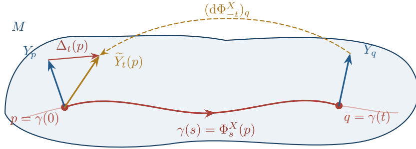
Rysunek 2.4: Punkty p = \gamma(0) i q = \gamma(t) = \Phi_t^X(p) leżą na tej samej krzywej całkowej na M ; czerwona strzałka pokazuje ruch w czasie od p do q . Wektor Y_q cofamy różniczką przepływu do T_pM , otrzymując \tilde{Y}_t(p) . Tam porównujemy go z Y_p ; \Delta_t(p) jest ich różnicą. Przerywana strzałka przedstawia transport wektora, nie ruch punktu.
