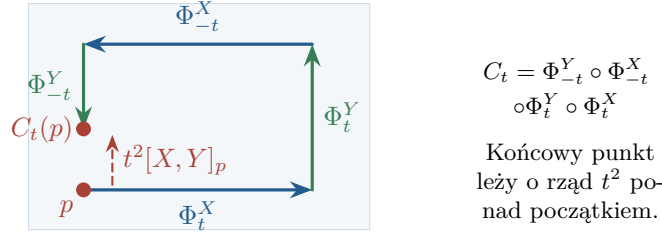
Rysunek 2.1: Komutator małych przepływów. Po przejściu kolejno wzdłuż X, Y, -X, -Y droga zwykle się nie zamyka; pierwsze niezerowe przemieszczenie wskazuje nawias [X, Y] . Rysunek ilustruje przykład X = \partial_x, Y = (1+x)\partial_y .
