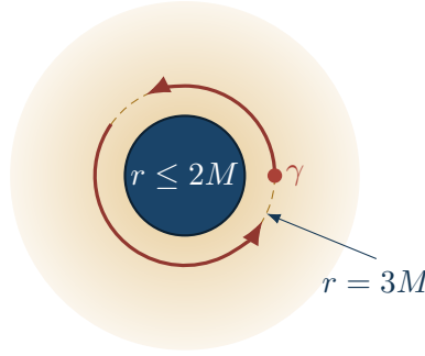
Rysunek 12.7: Schemat rzutu na współrzędne (r, \phi) równikowej geodezyjnej światłopodobnej Schwarzschilda o stałym r = 3M . Ciemny dysk oznacza r \leq 2M w tym rysunku współrzędnych; okrąg r = 3M nie przedstawia geodezyjnej metryki indukowanej na przekroju przestrzennym.
