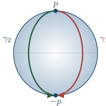
Rysunek 12.3: Dwa różne półokręgi wielkich kół łączą p z antypodą. Każdy ma długość \pi R . Rysunek jest rzutem ortogonalnym: półokręgi widać jako połówki elips, a równik jako odcinek. Przedłużenie łuku za antypodę nie minimalizuje już długości od p .
