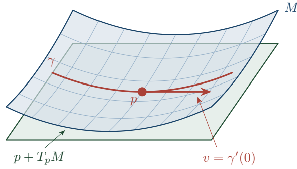
Rysunek 1.8: Przestrzeń styczna: zielony równoległobok przedstawia afiniczną płaszczyznę p + T_p M przy osadzonej powierzchni M . Czerwona krzywa \gamma leży na M , a wektor v = \gamma'(0) leży w płaszczyźnie stycznej. Siatka powierzchni odchyła się od tej płaszczyzny poza punktem p .
