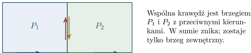
Rysunek 9.3: Znak orientacji usuwa wewnętrzną krawędź przy składaniu dwóch fragmentów.
