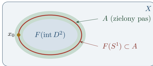
Rysunek 8.2: Przykład odwzorowania względnego (D^2, S^1, *) \rightarrow (X, A, x_0) . Czerwony obraz brzegu leży w zielonym pasie A , podczas gdy obraz wnętrza dysku może wyjść poza A . W ogólnej definicji nie wymaga się różnowartościowości F .
