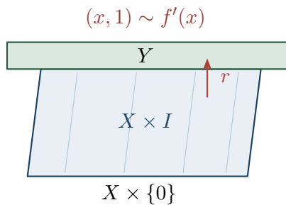
Rysunek 8.3: Cylinder odwzorowania zamienia odwzorowanie f' : X \rightarrow Y na włączenie podkompleksu X \hookrightarrow M_{f'} . Rysunek pokazuje mechanizm dowodu twierdzenia Whiteheada.
