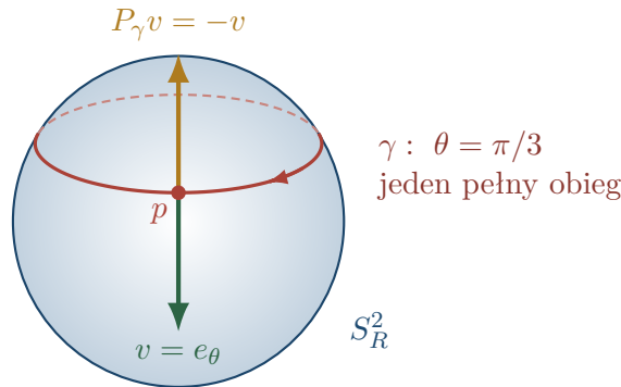
Rysunek 11.2: Transport po równoleżniku \theta = \pi/3 obraca wektor o -\pi . Dla czytelności początek pętli wybrano w punkcie p o \phi = \pi/2 (zakres parametru przesuwają się wtedy o \pi/2 ). Strzałki są rzutami przeciwnych wektorów w tej samej płaszczyźnie T_p S_R^2 , narysowanymi w tej samej skali. Przerywana część równoleżnika leży z tyłu sfery.
