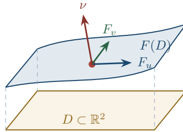
Rysunek 10.2: Parametryzacja unosi obszar parametrów D na powierzchnię. Wektory F_u, F_v wyznaczają element pola \sqrt{\det(g(F_u, F_v))} du dv ; normalna \nu pozwala dodatkowo mierzyć strumień.
