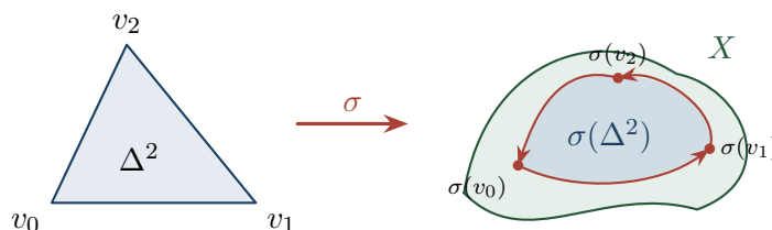
Rysunek 7.2: Singularny sympleks jest odwzorowaniem do X , niekoniecznie płaskim trójkątem. Jego brzeg liczymy z ograniczeń odwzorowania \sigma do trzech ścian.
