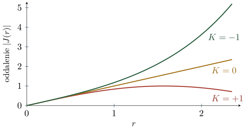
Rysunek 13.6: W modelach o krzywiznach +1, 0, -1 zerowe początkowe wychylenie i jednostkowa pochodna D_r J(0) dają odpowiednio |J(r)| = \sin r, r, \sinh r . Wykres pokazuje zakres 0 \leq r \leq 2,35 ; pierwsze ponowne zero na sferze występuje później, przy r = \pi .
