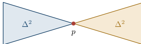
Rysunek 9.5: Dwa trójkąty ze wspólnym wierzchołkiem p . To kompleks symplecjonalny, ale w p nie jest powierzchnią gładką, nawet z brzegiem.
