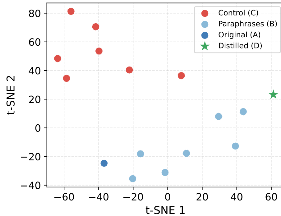
Layer 16
