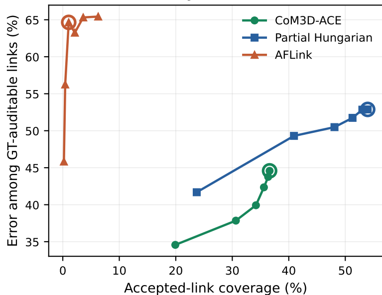
ByteTrack
