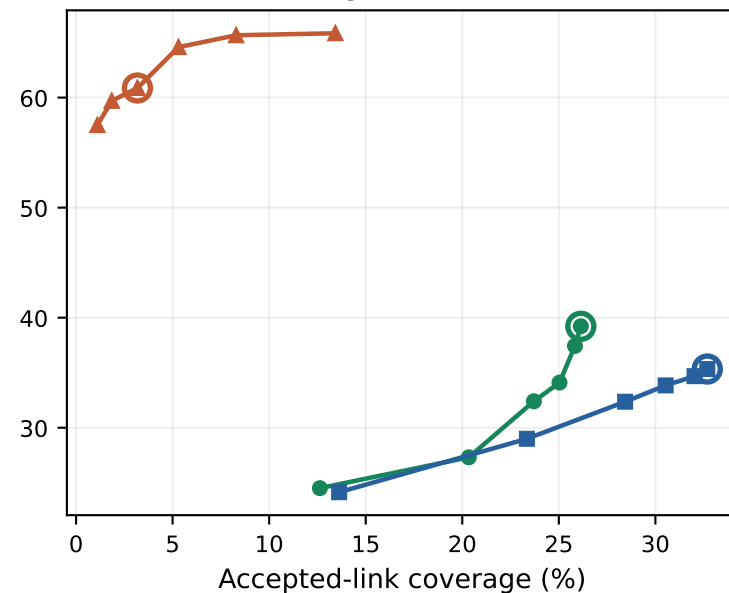
Deep OC-SORT
