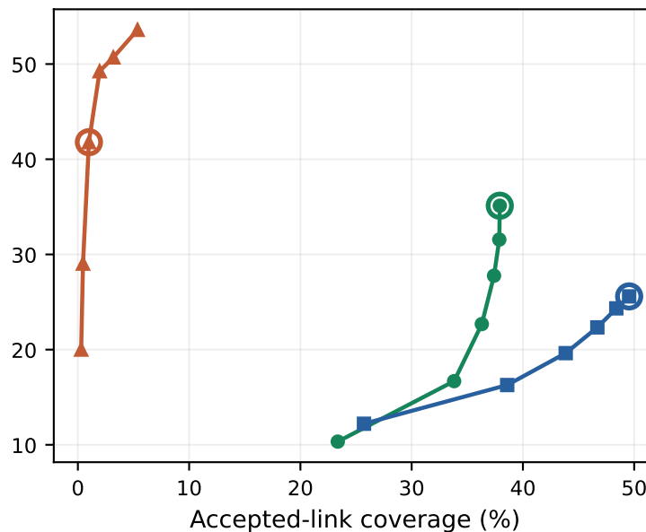
OC-SORT
