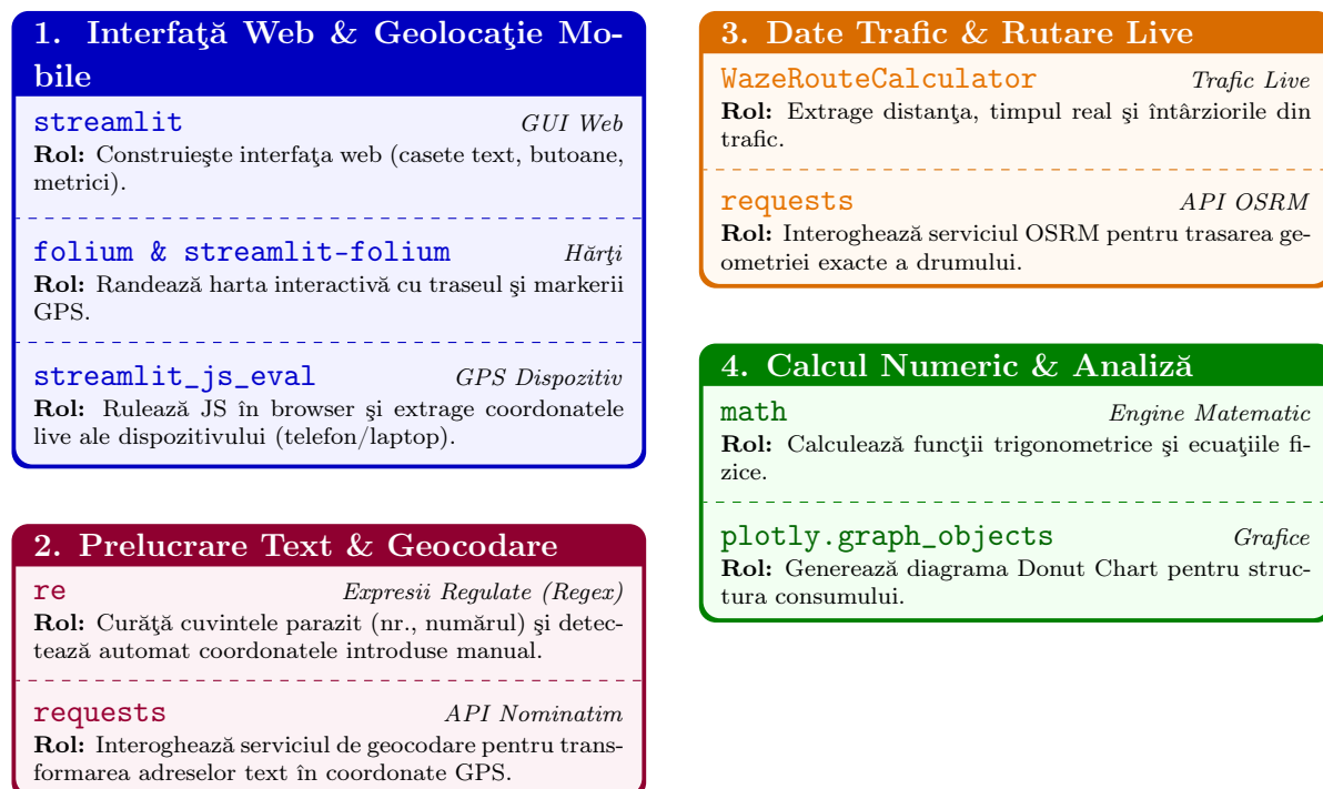
Figura 2: Structura modulară extinsă a bibliotecilor Python utilizate în aplicație.
