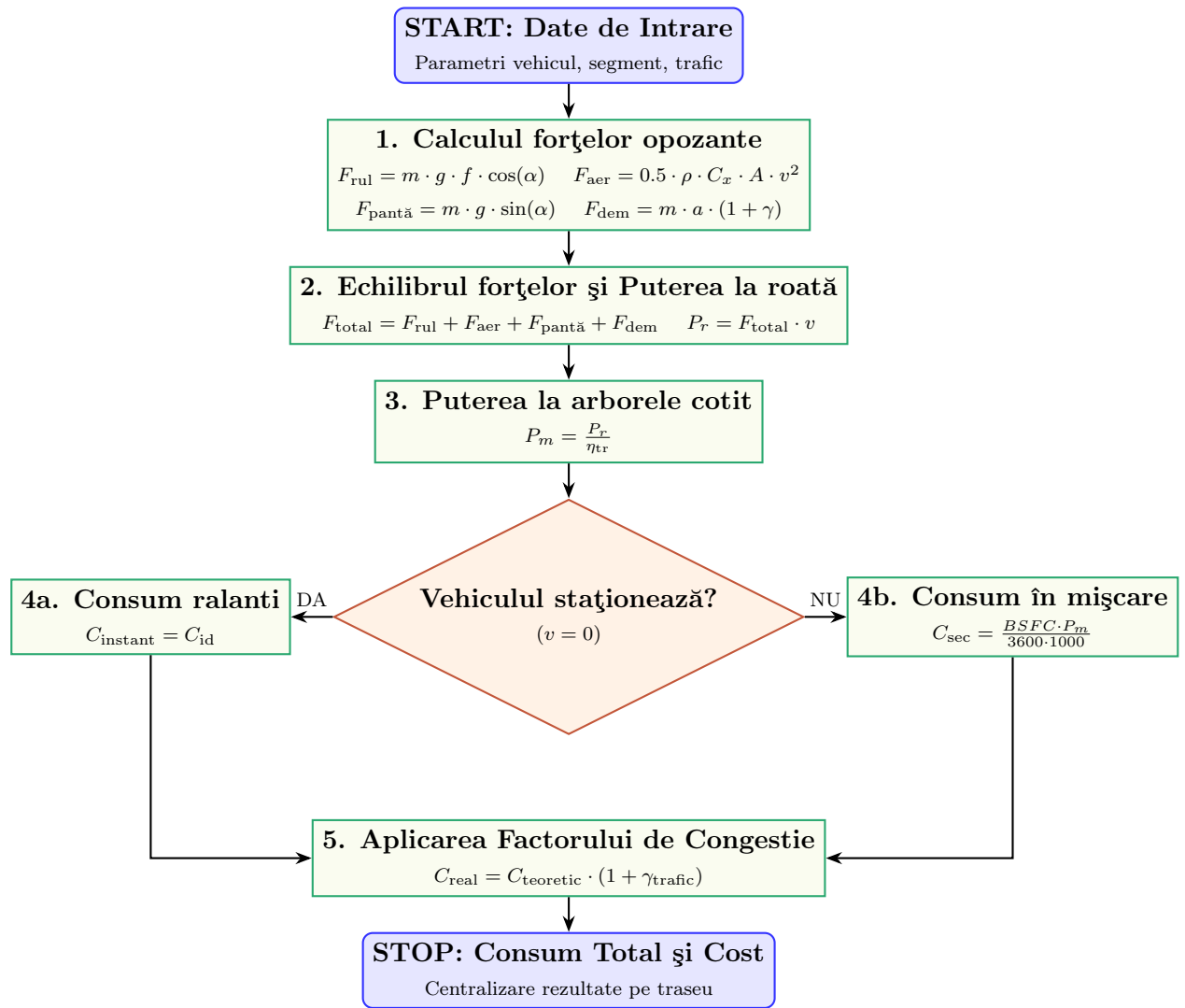
Figura 1: Schema fluxului matematic pentru modelarea consumului de combustibil.
