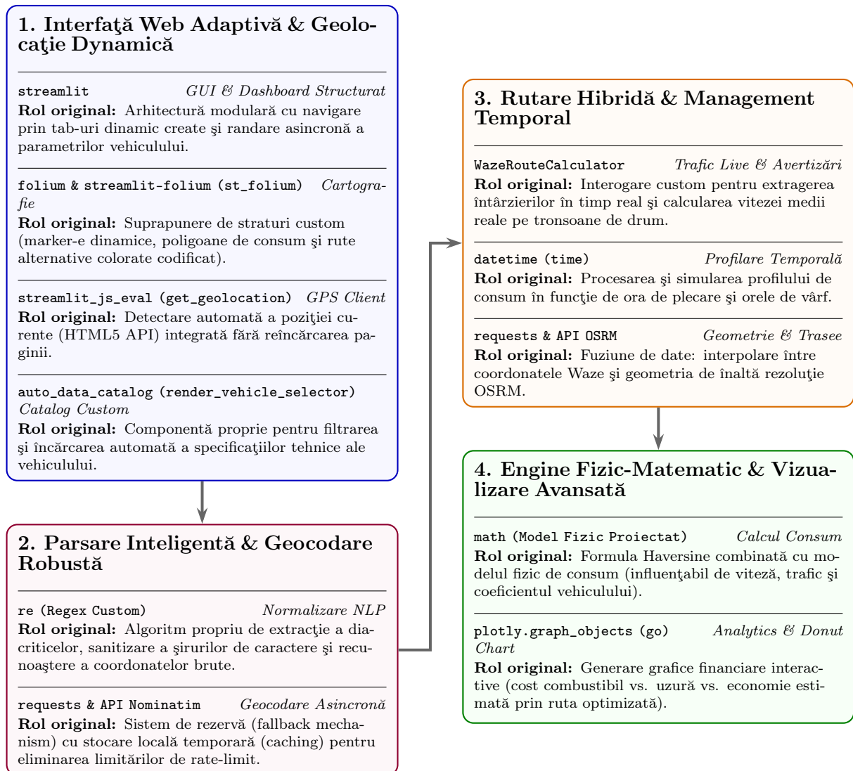
Figura 2: Bibliotecile utilizate în cadrul dezvoltării aplicației Python.
