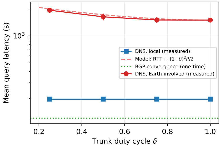
(b) Mars ( P = 1800 s)
