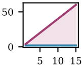
(c) Mars
