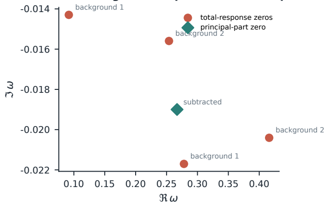
(d) Background-dependent total-response zeros
