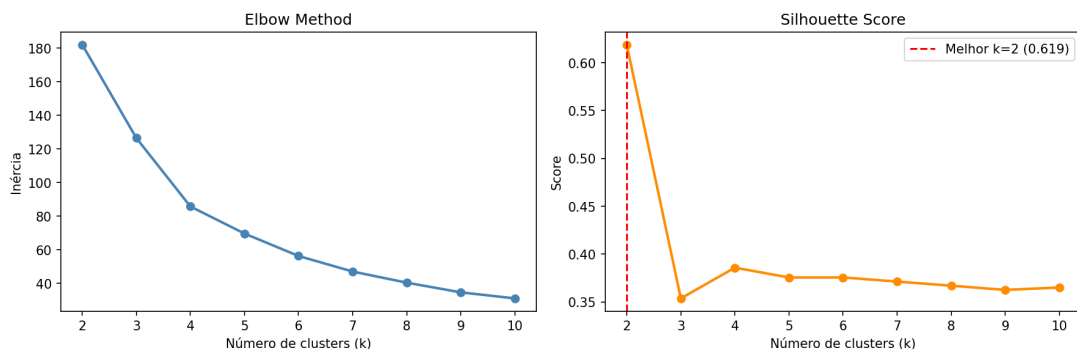
Figura 2 – Curvas de inércia (esquerda) e Silhouette Score (direita) para k \in \{2, \dots, 10\} . A linha vertical vermelha indica o k ótimo segundo o silhouette.
