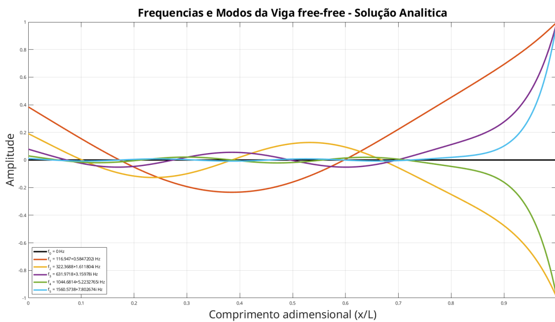
Figura 8 – Formas modais da viga livre-livre
