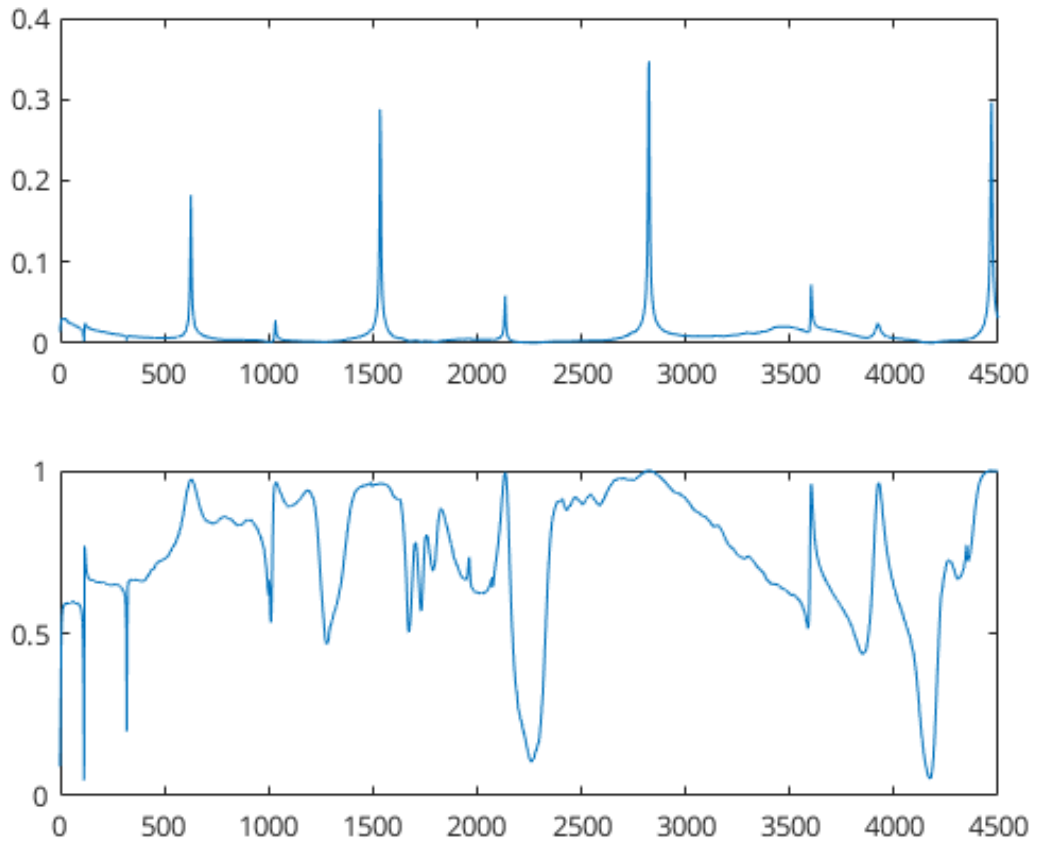
Figura 5 – FRF e coerência experimental
