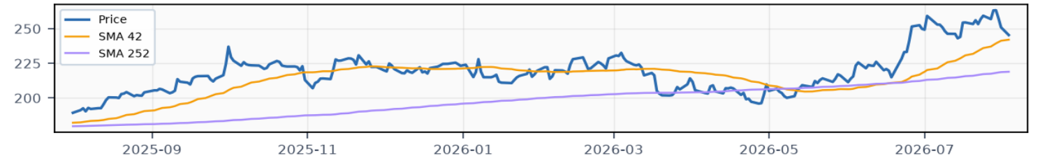
ABBV · Price & SMA
