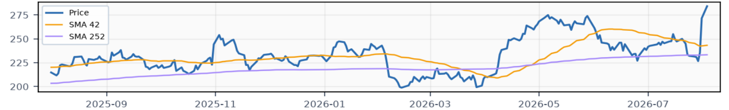
AMZN · Price & SMA
