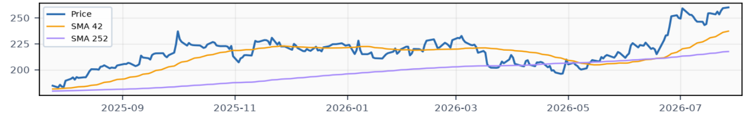
ABBV · Price & SMA
