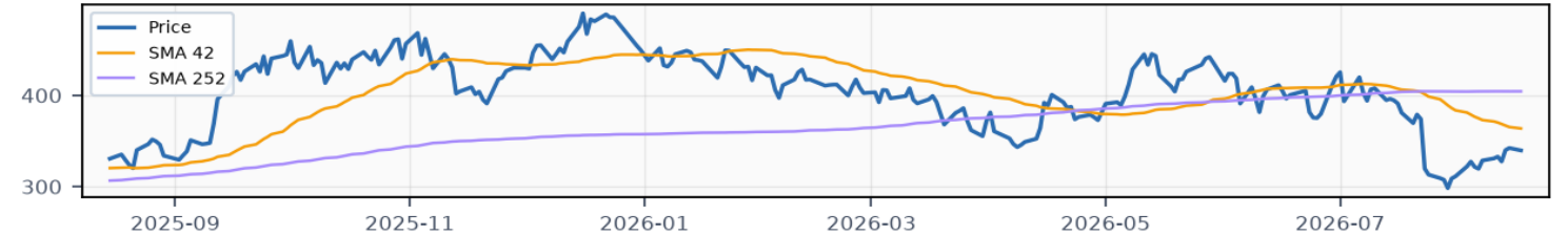
TSLA · Price & SMA
