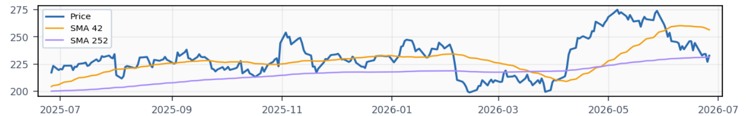
AMZN · Price & SMA
